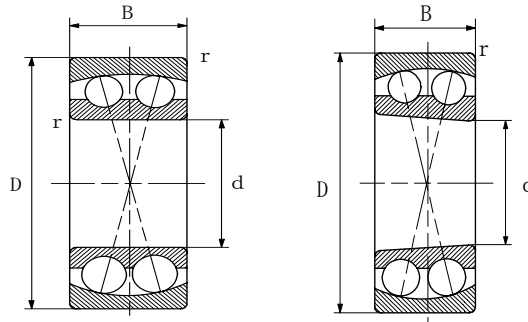
円筒穴
