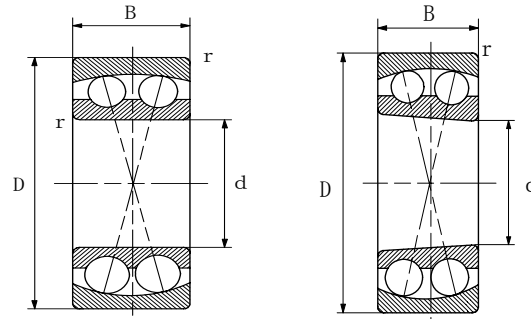
円筒穴
